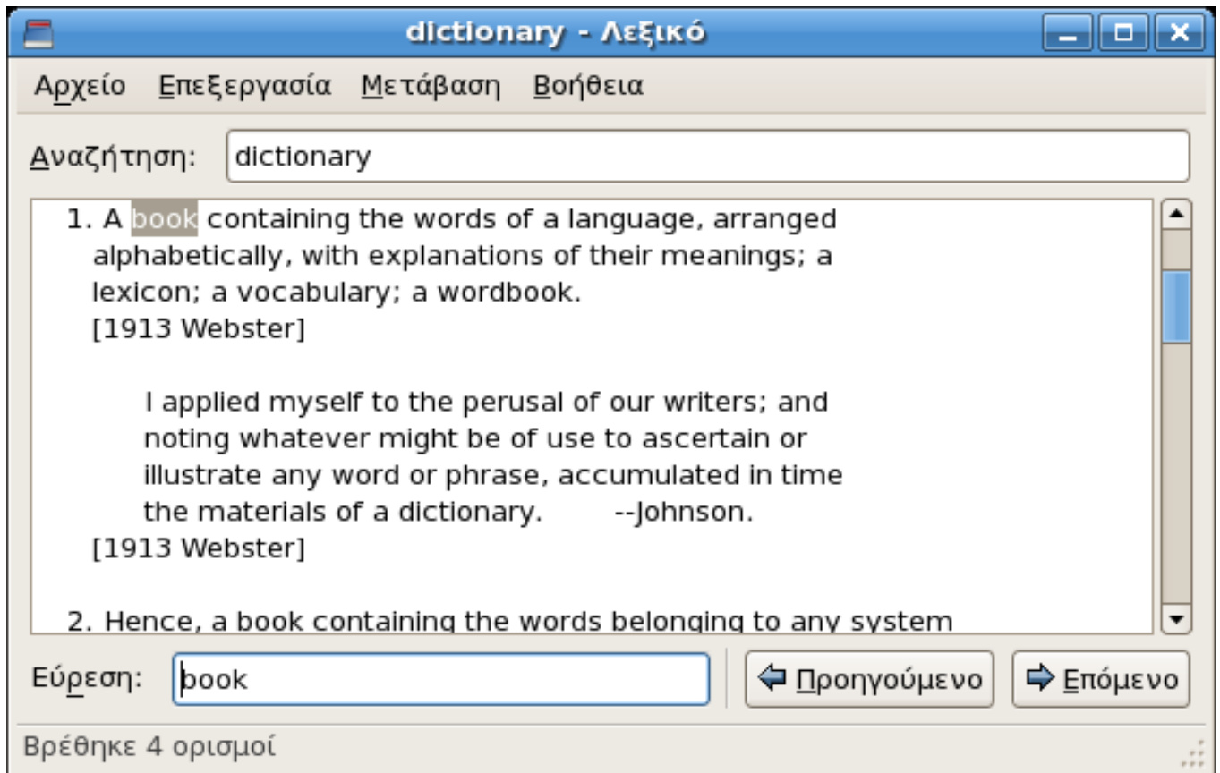
Figure 3: Παράθυρο λεξικού
