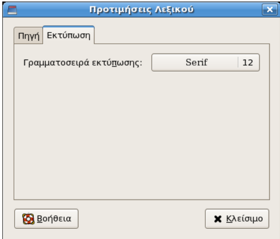
Figure 6: Παράθυρο λεξικού
